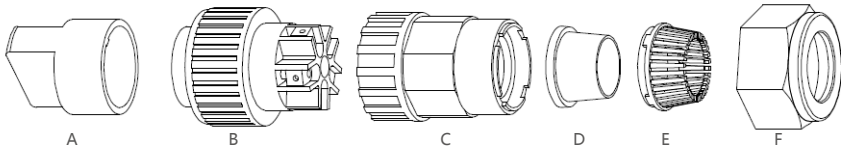
Figura 5.19 Conector de CA
