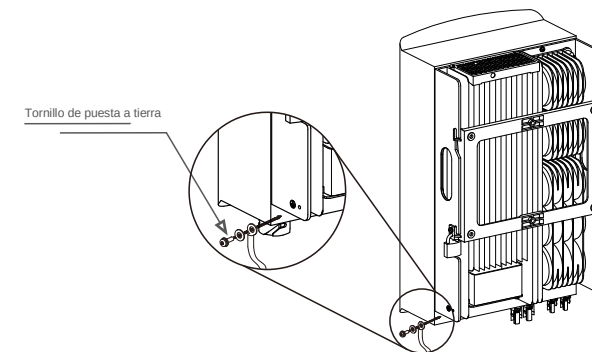
Figura 5.10 Cable fijo
