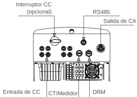
Figura 1.2 Vista inferior
