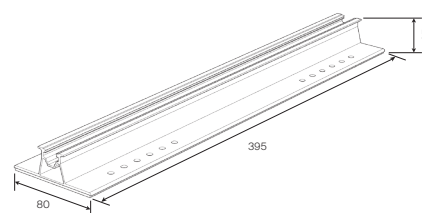
Halterung für Hochformatmontage (mm)
