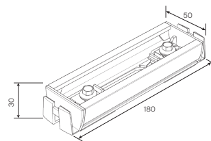
Halterung für Querformatmontage (mm)
