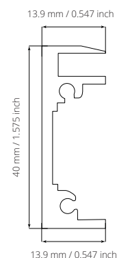
Frame doorsnede
